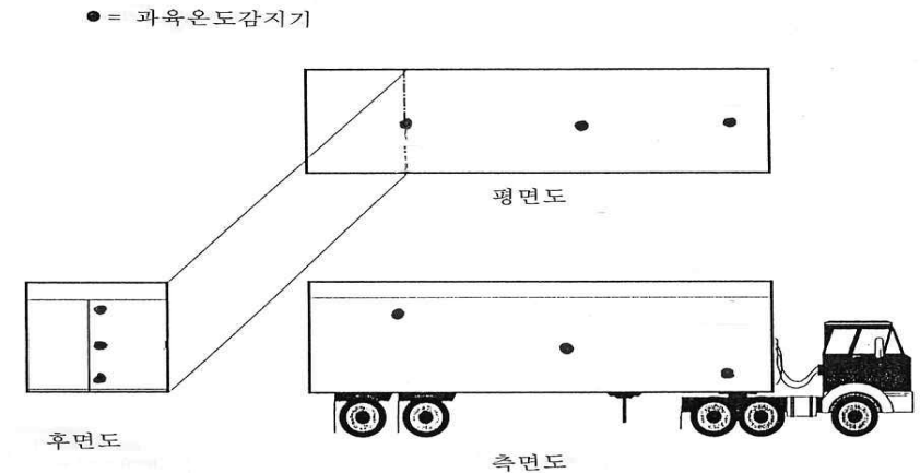
[그림 1.] 수송 중 저온처리시 과일 중심부 온도 측정을 위한 온도센서의 위치
